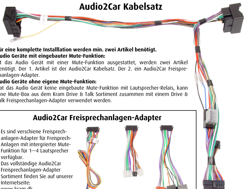
Beispiele div. Freisprechanlagen Adapter
