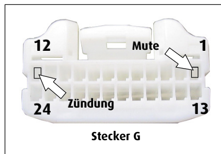
Abb.: 24-pol. Steckverbinder am Verstärker
