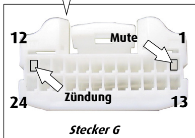
Abb.: 24-poliger Stecker am Verstärker
