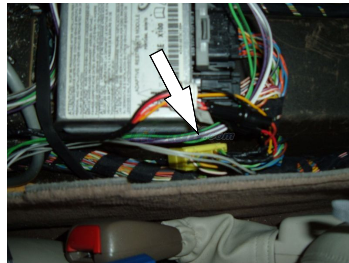
Abb.: Position des 10-pol. VDA Steckverbinders in der Mittelkonsole
