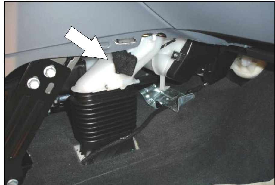
Foto: Position des VDA Konnektors im Saab 9.3 Sport.
